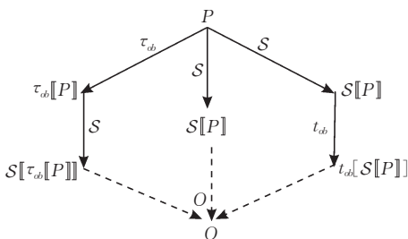
图 1 迷惑算法的正确性关系
